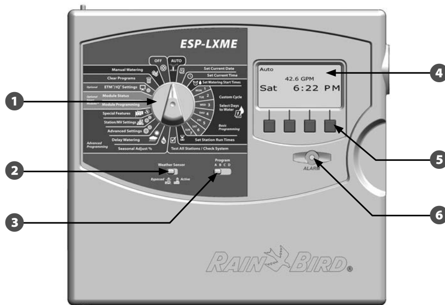
Элементы передней панели контроллера ESP-LXME
