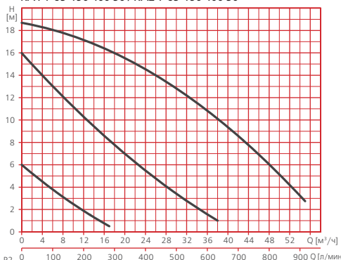
RA1-F 65-190 400 50 / RA2-F 65-190 400 50
