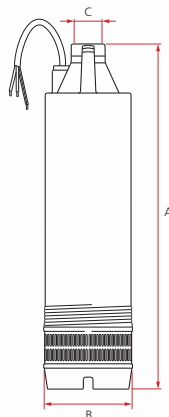
ACUARIA37 / ACUARIA57
