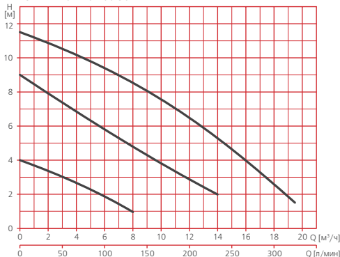
RSAN-F 40-120 400 50
