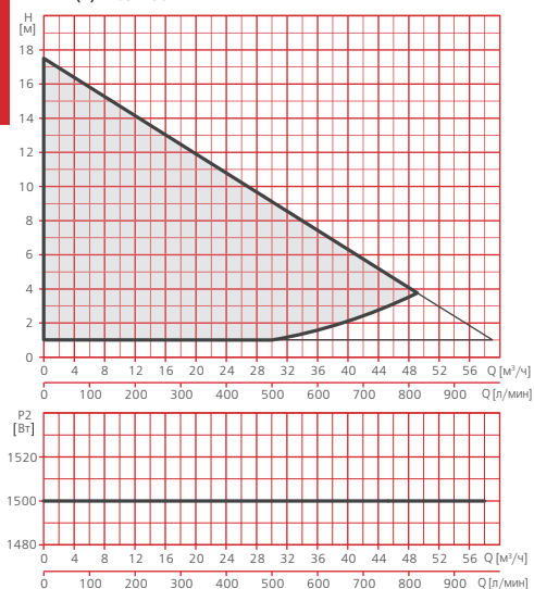
RV1(2)-F 65-180
